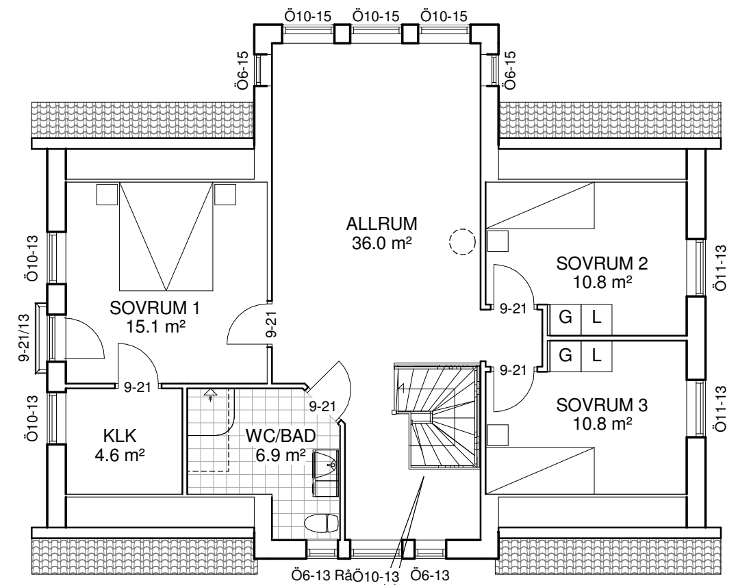
Övervåning
